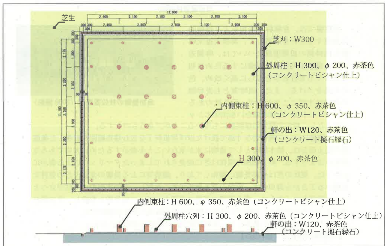
Ⅲ期 (SB37) 柱表示 平面図・断面図 (S=1/200)
