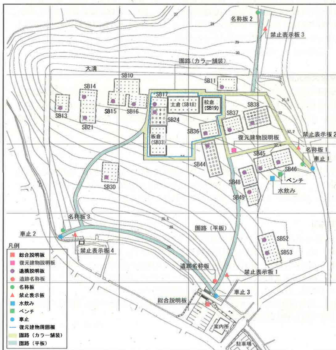
現状全体配置図 1:1600
