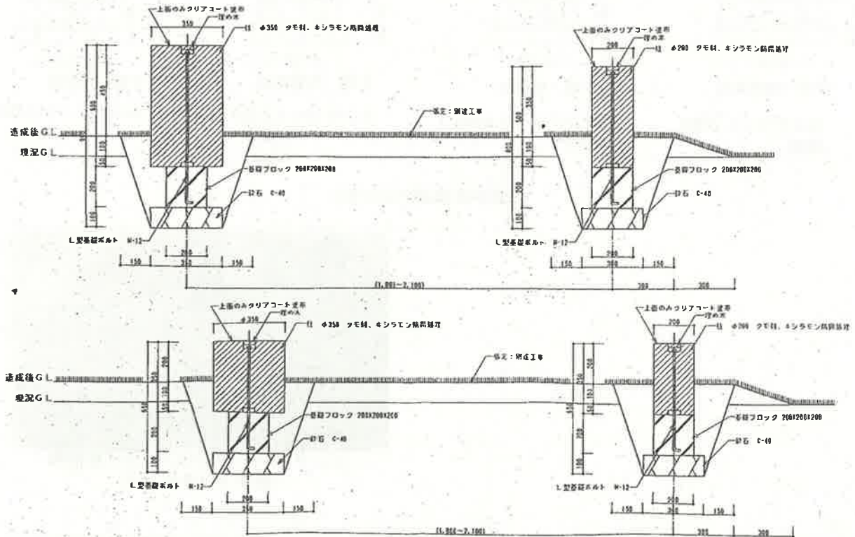
当初整備詳細図
