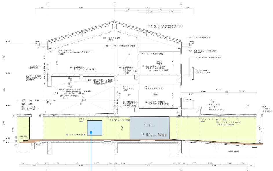
アートゲート断面図
