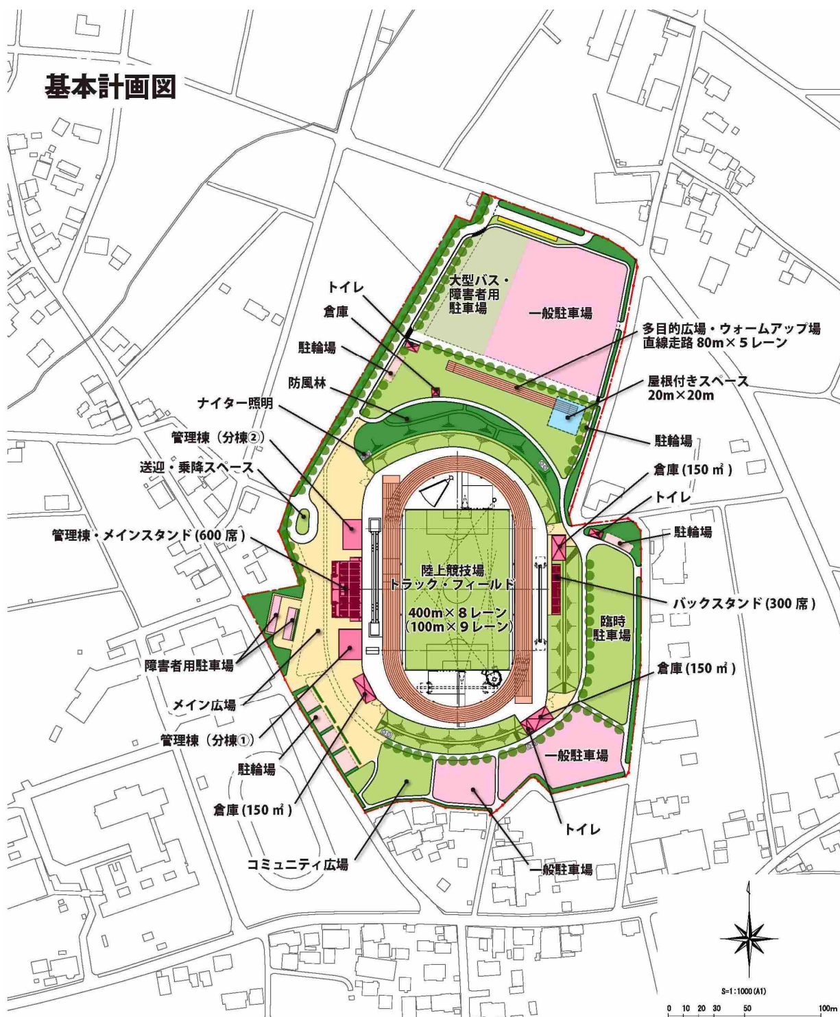
図 3-12 基本計画図
