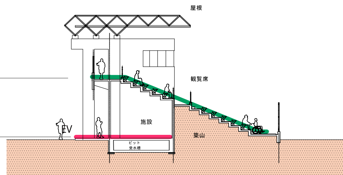
断面計画
