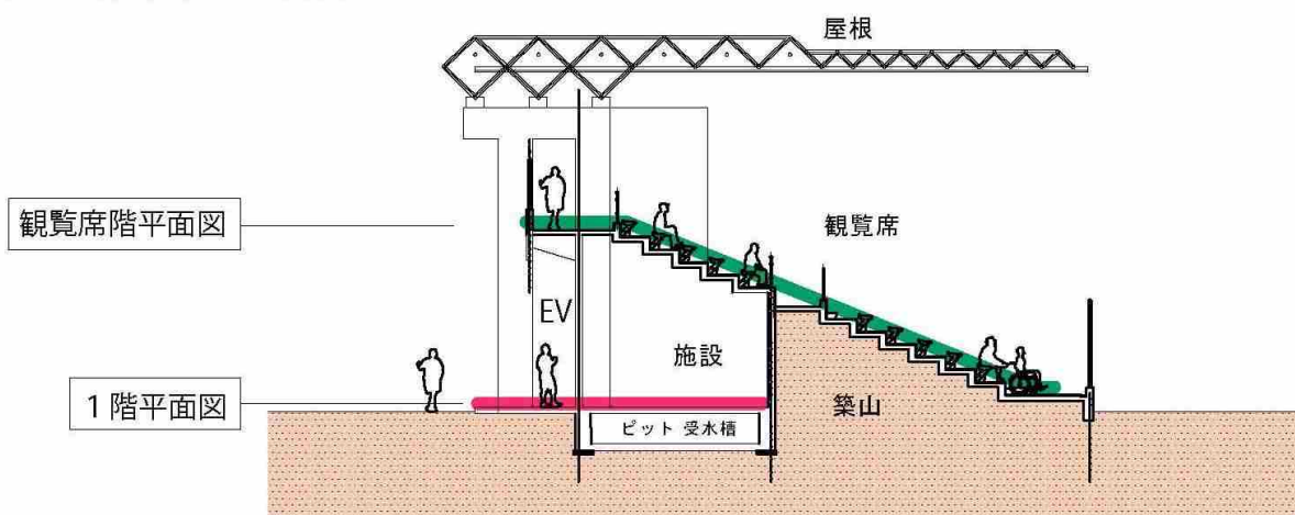
図 3-14 管理棟・メインスタンド平面・断面図
