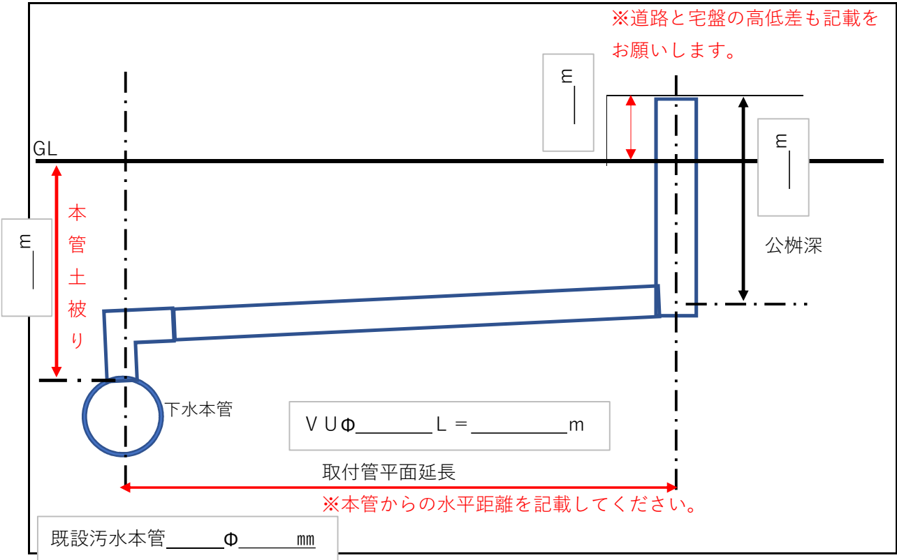
断面図
