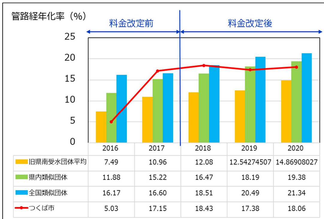
図 2-15 経年化率
