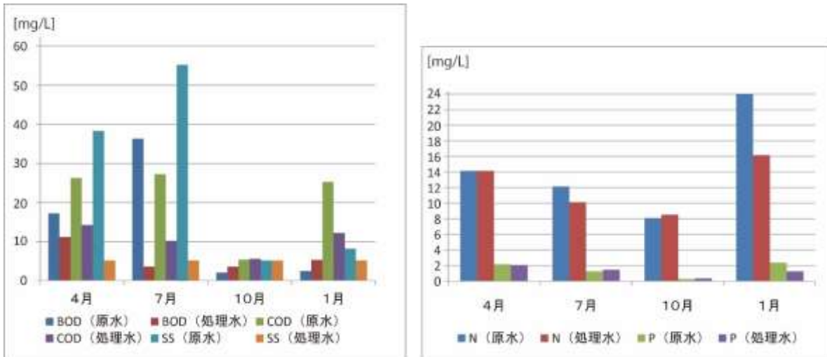
図表 2 - 1 - 13 上菅間地区生活排水路浄化施設水質調査結果
