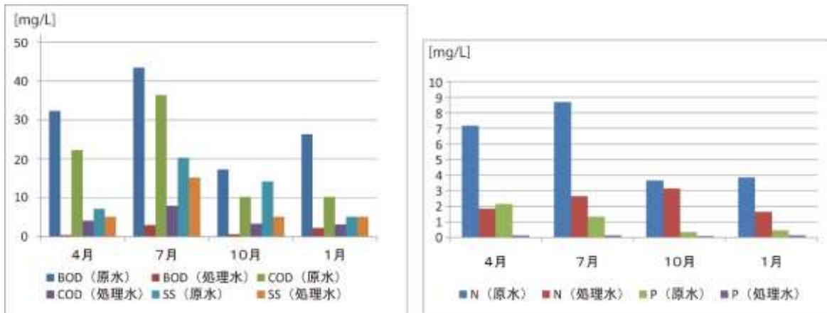
図表 2 - 1 - 14 佐地区生活排水路浄化施設水質調査結果
