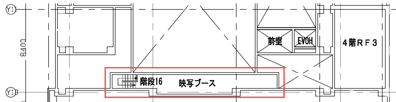
4 階平面図
