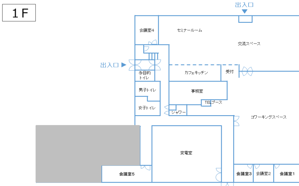
(9)建物平面図
